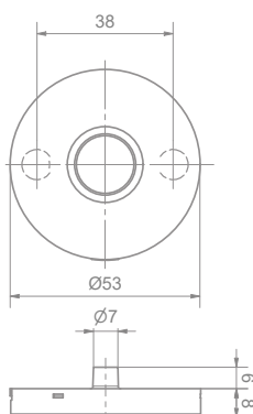
Topaz 5632C Rosaces de poignée
